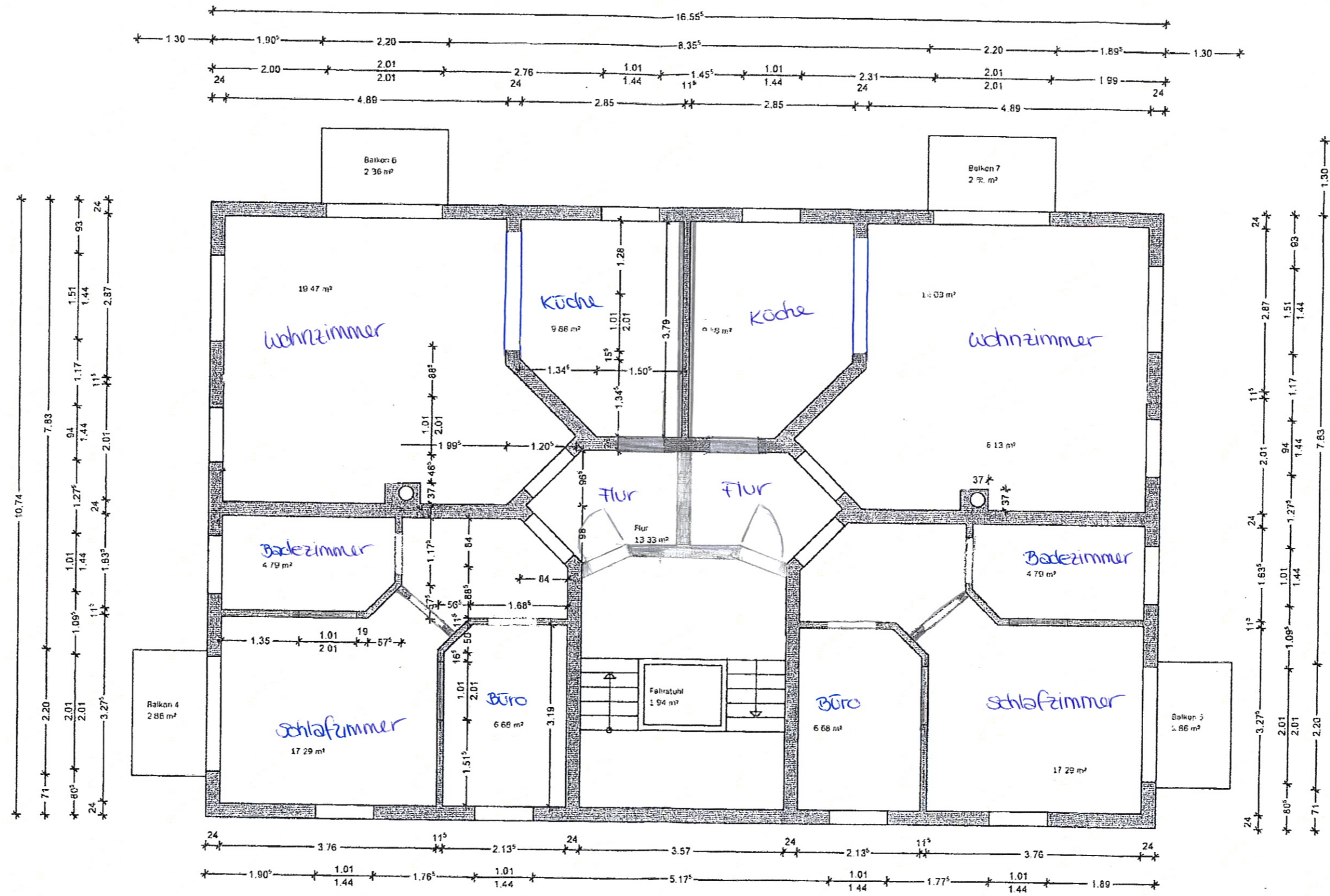
Obergeschoss
